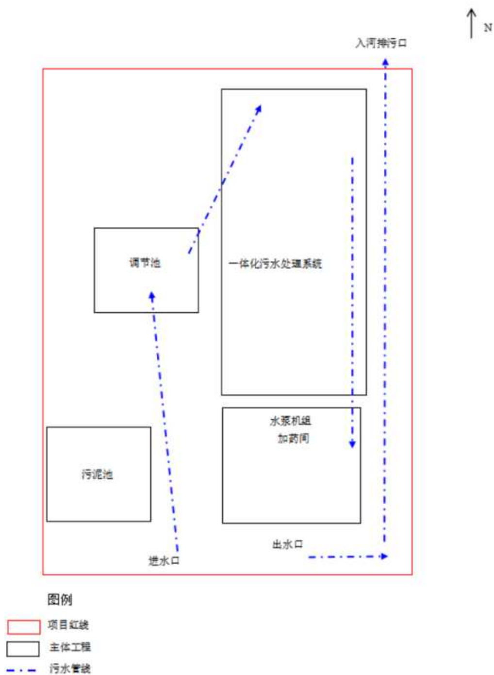
（白坑村 B 区污水处理站）
