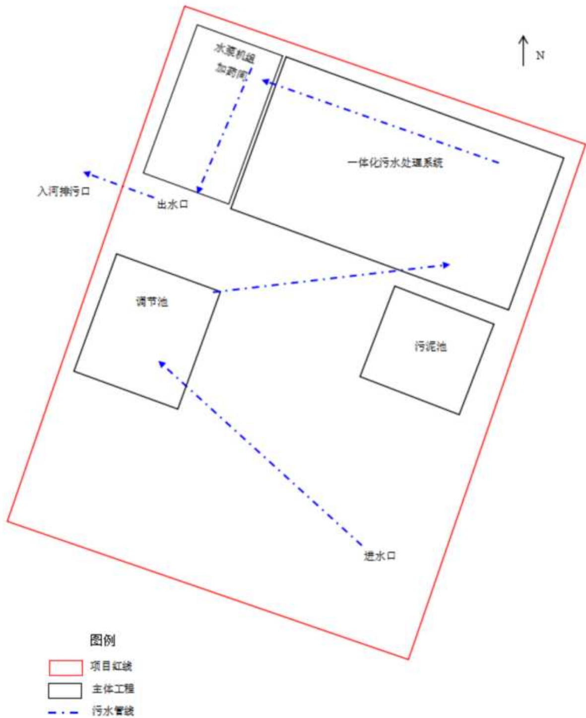
(红星村A区污水处理站)
