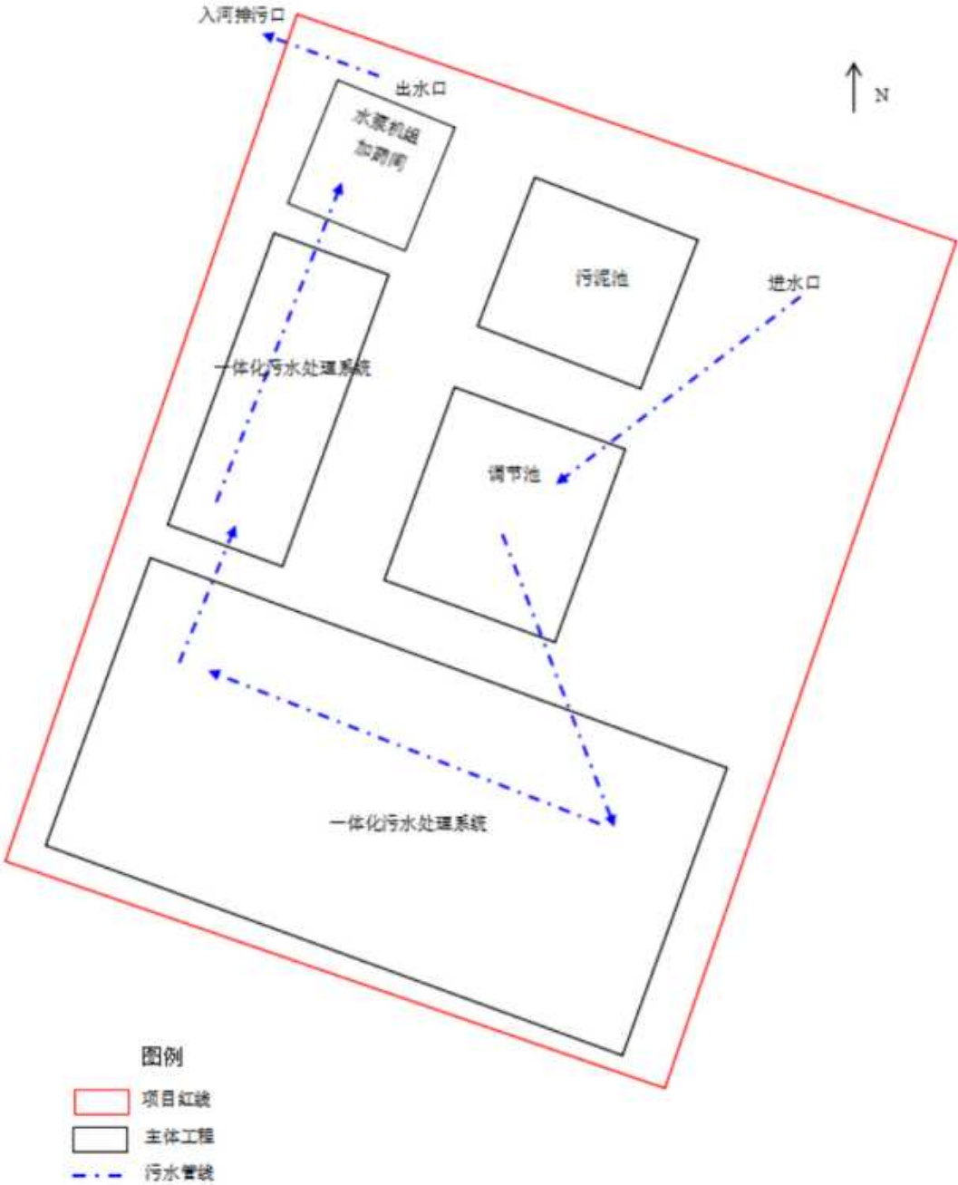
（新厝村污水处理站）
