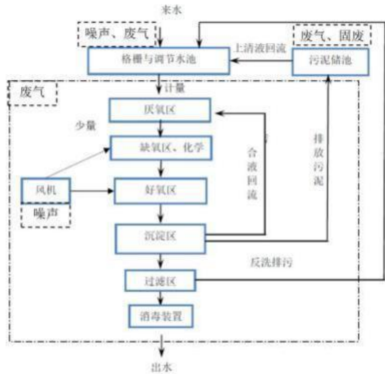
图 2-1 污水处理站生产工艺流程图及产污环节
